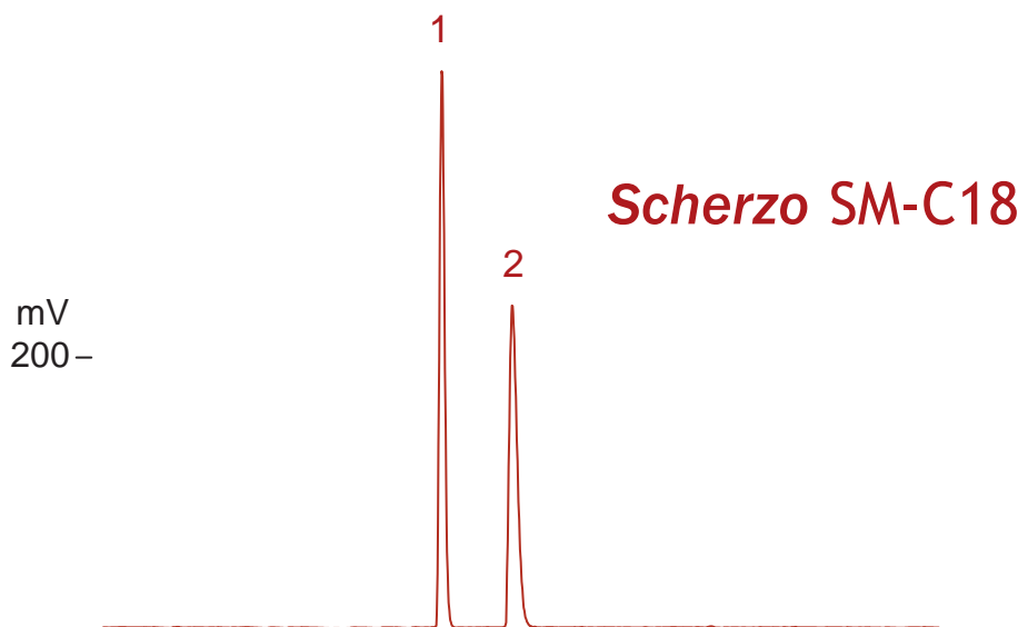
DL-mevalonolactone
