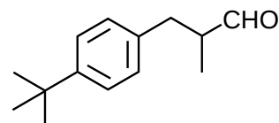
3-(4-tert-butylphenyl) -2-methylpropanal
